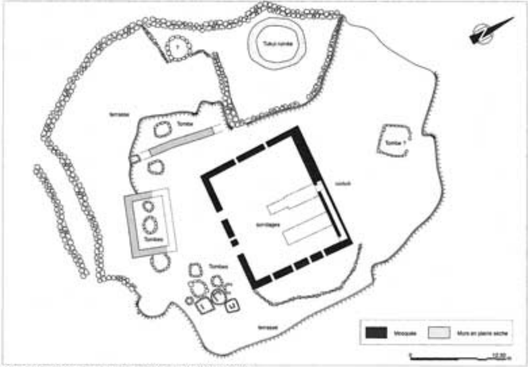
Mosquée de Fâqj Dâbbis - Plan général (Dessin : Régis Bernard - AFAN, Mars 2006)
